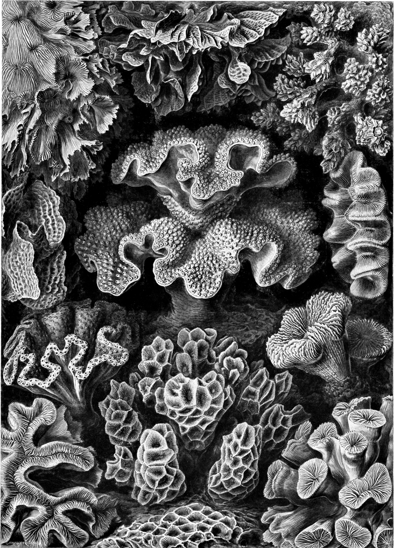
Hexacoralla. — Sechsstrahlige Sternkorallen.
